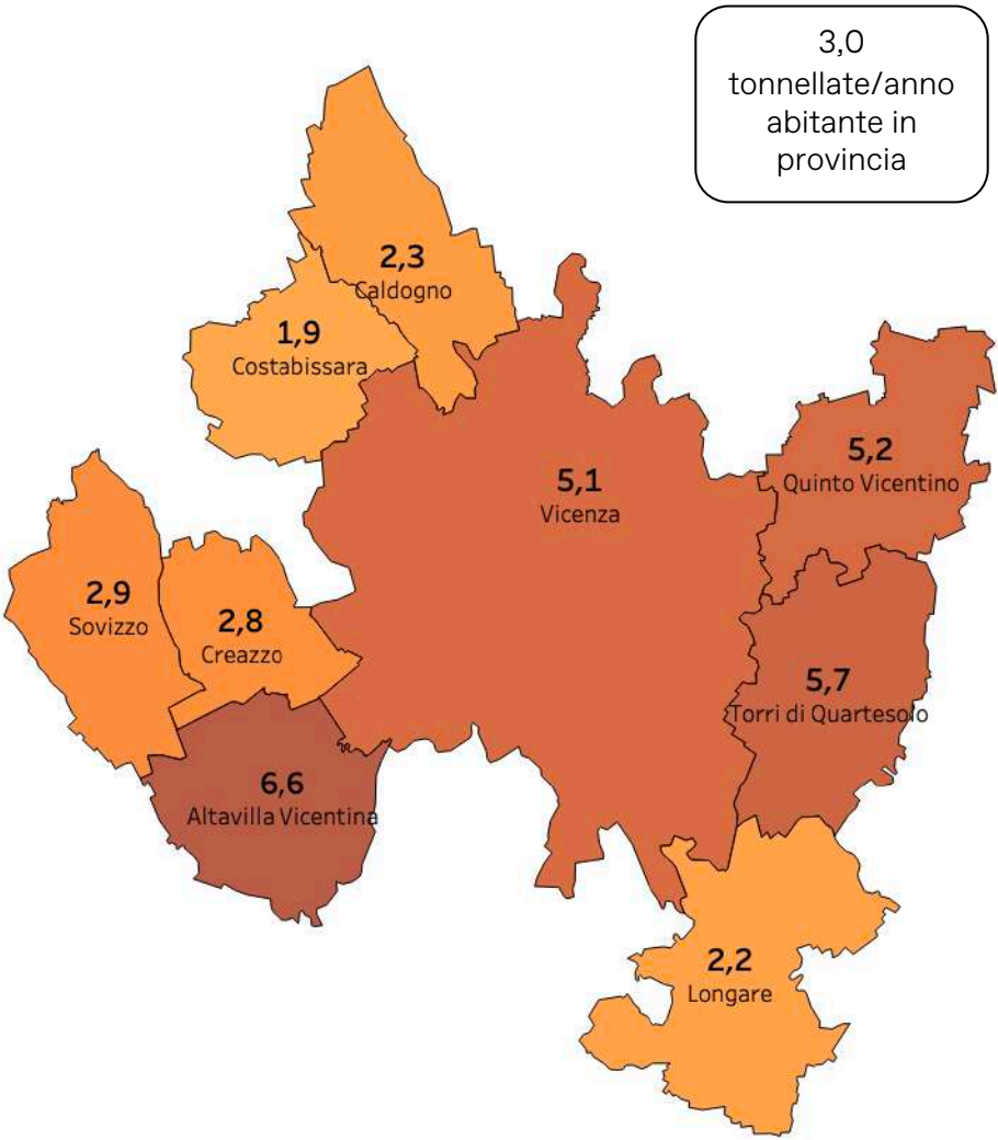
Tonnellate di CO2 prodotte/anno ad abitante
