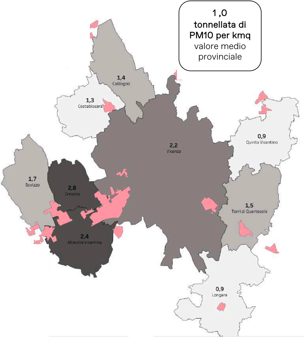
Produzione tonnellate/anno di PM10 per kmq
